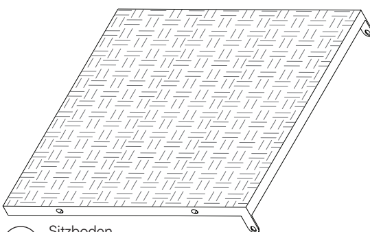
4 Sitzboden 2x
